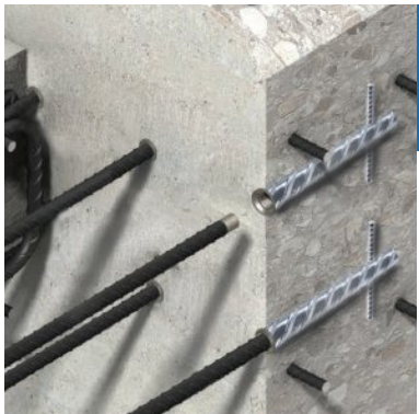
PRECAST CONCRETE LIFTING & CONNECTING SYSTEM PHỤ KIỆN NÂNG CẦU & KẾT NỐI CẤU KIỆN BÊ TÔNG
